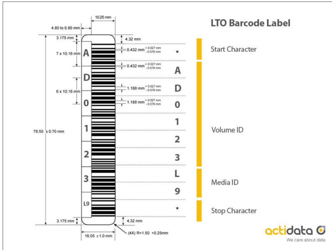
Abmessungen und Kodierung LTO-Medium (LTO-Datenkassette)
